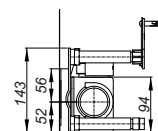
drain body DallFlex
